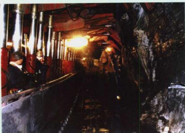
铁煤集团依靠科技进步，提高装备档次，综采机械化程度已达 97.61%。图为日产 7000 吨的大兴矿综采工作面
