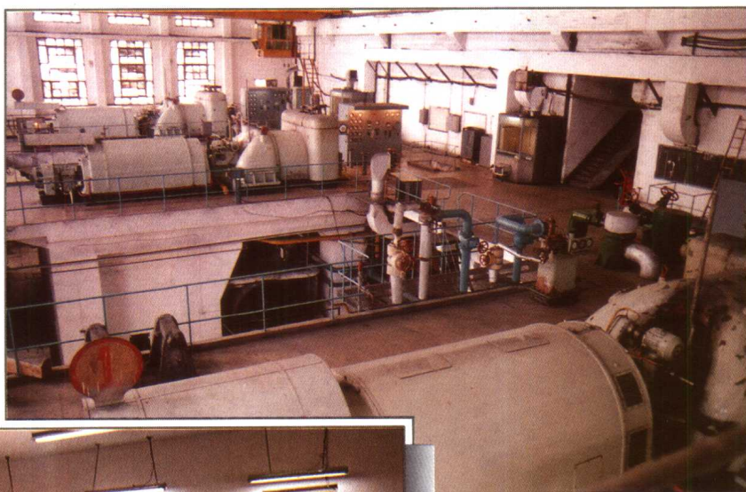
三台1.2万千瓦机组汽机房。
