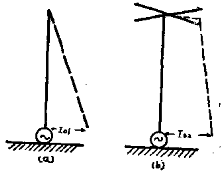
图3-5 加顶负载后改善了电流分布
