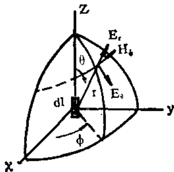
图2-3 电流元的坐标系
