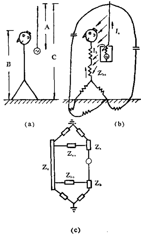
Z_c 操作者 Z_a 天线 Z_b 电台箱
