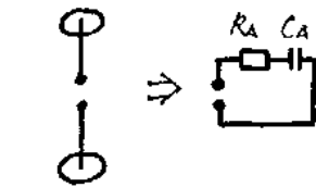
图 1-1 电容性天线的等效电路
