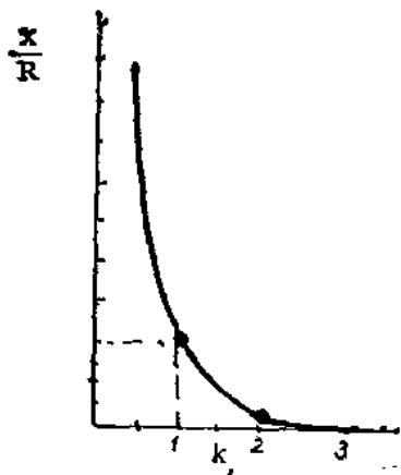
图2-5 \left| \frac{x}{R} \right| \sim kr 曲线
