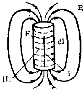
图2-1 电流元附近的场分布
