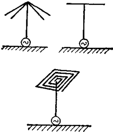
图3-4 各种加顶的鞭天线
