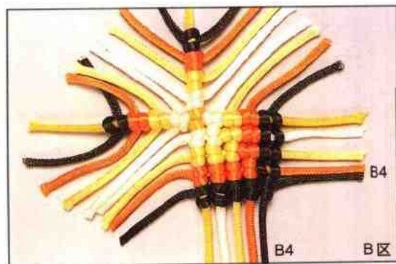
⑩ B区以右边B4为轴，以左边B4为编线，编斜卷结。
