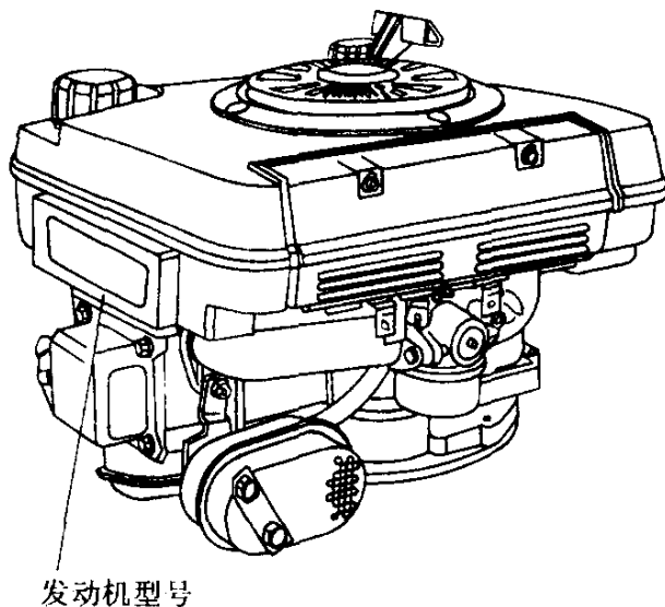
图 1-3 单缸风冷卧式四行程 小汽油机外形图
