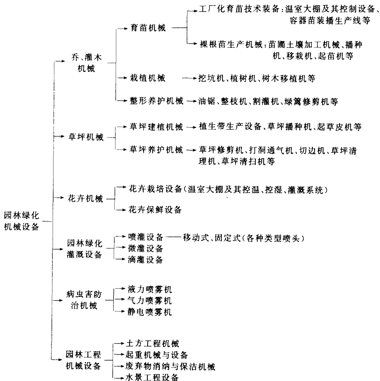
图 1-1 按作业对象和主要功能分类
