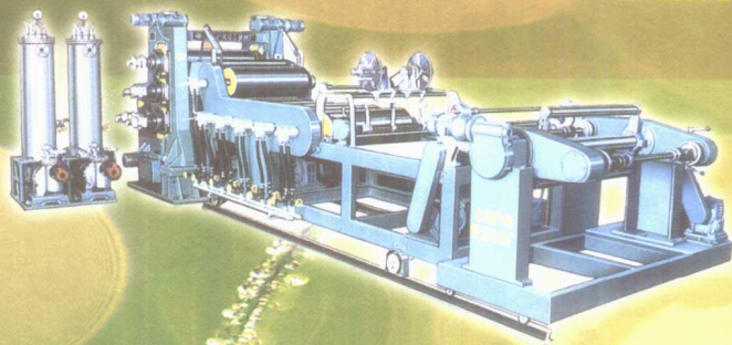
SY-F5L860 五辊压延机组
