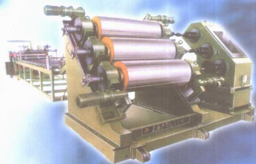
QDYG ~ 400X1400 斜式三辊压光机组
