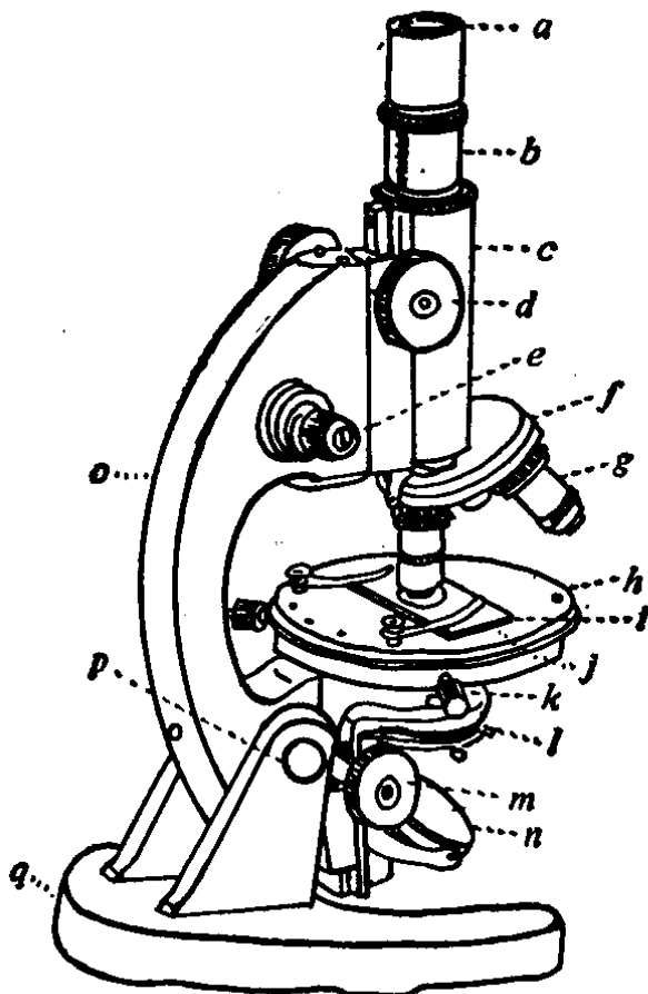
图 1-1 中级显微镜的外形和各部分名称
