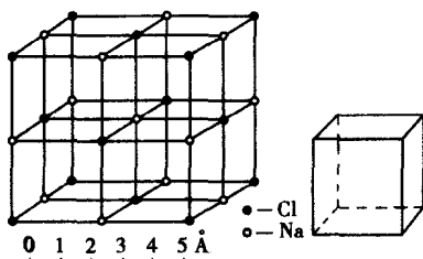
图1.1.1 岩盐的内部结构和晶体
