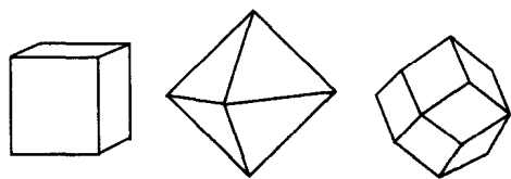
图1.1.2 矿物的几种外形
