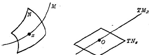
图2 子流形的切空间
