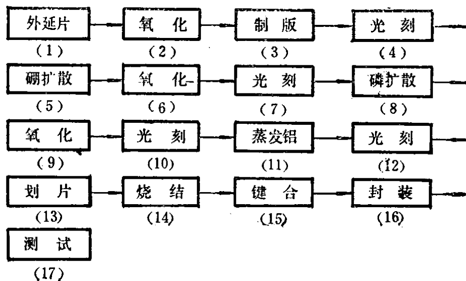
图 1-1 平面晶体管的工艺过程
