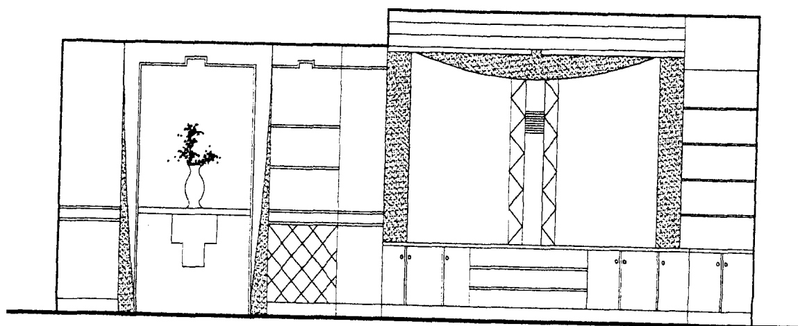
立面图
