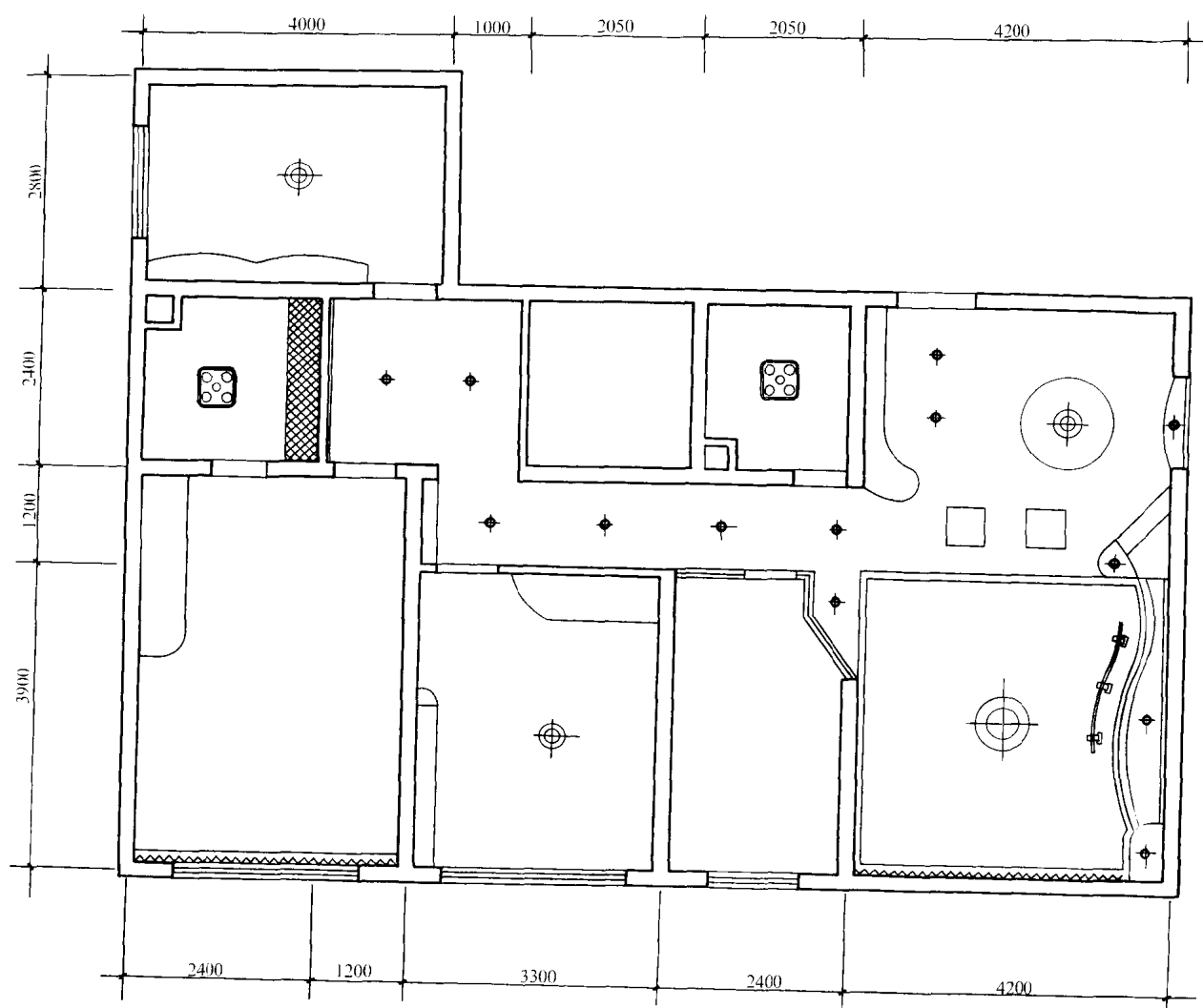
顶棚平面图
