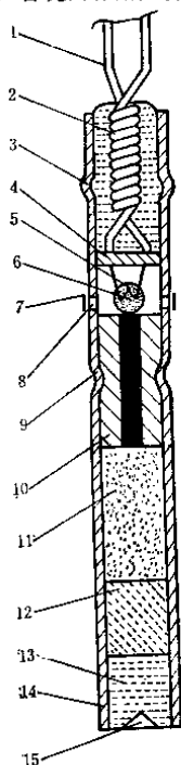
图1-5 延期电雷管
