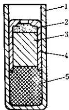
图1-3 针刺雷管
