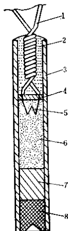
图1-4 瞬发电雷管
