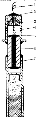
图1-2 拉发雷管
