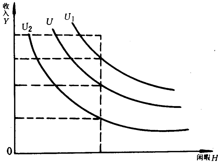
图 1—1 无差别曲线
