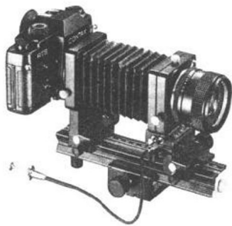
图 11B 近摄皮腔
