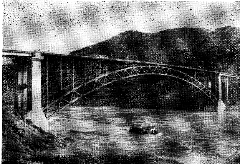
四川省金沙江上的一座钢拱桥，跨径 180 米
