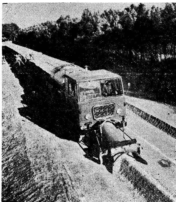
黑龙江省青冈县 自制的渣油路面 联合铺路机
