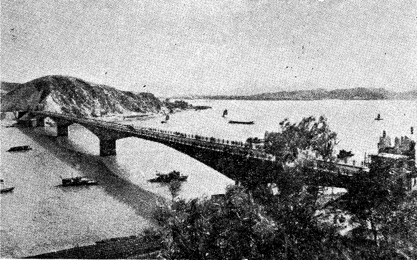
福建省乌龙江大桥，是一座预应力混凝土T型刚构桥，中部三孔为跨径144米，两边空各为58米。总长548米。采用悬臂拼装和悬臂浇注施工
