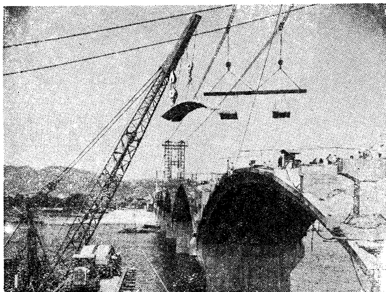
湘江大桥正在吊装腹拱拱圈
