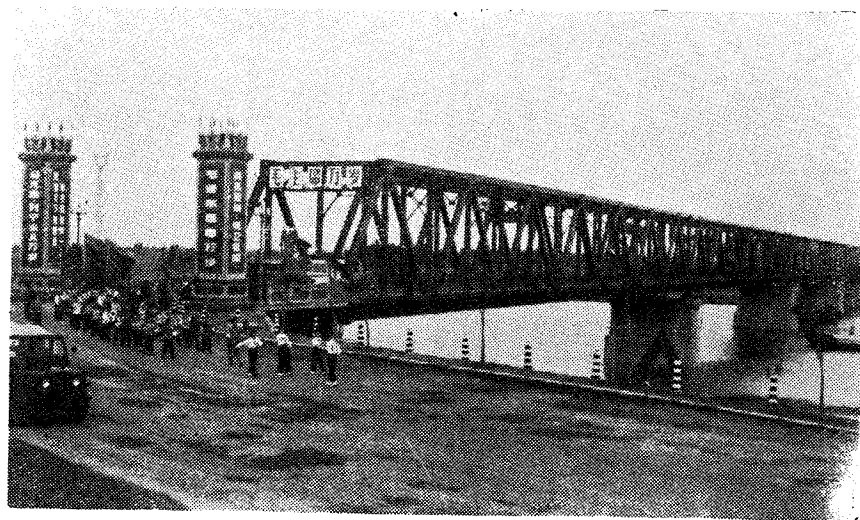
山东省北镇黄河大桥，主孔四孔为跨径 112 米栓焊连续钢桁架，边孔为钢筋混凝土梁式桥，全长 1391 米
