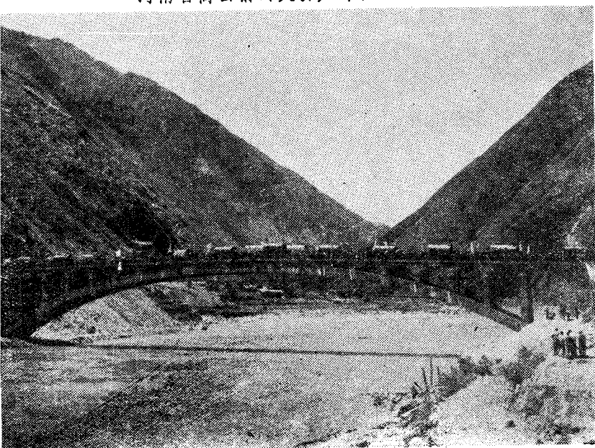
四川省泸定桥，单孔跨径 110 米的双曲拱桥
