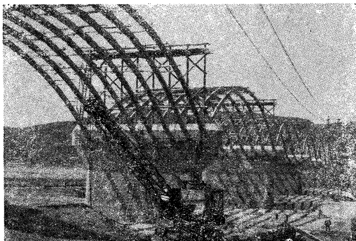
湘江大桥拱肋架装
