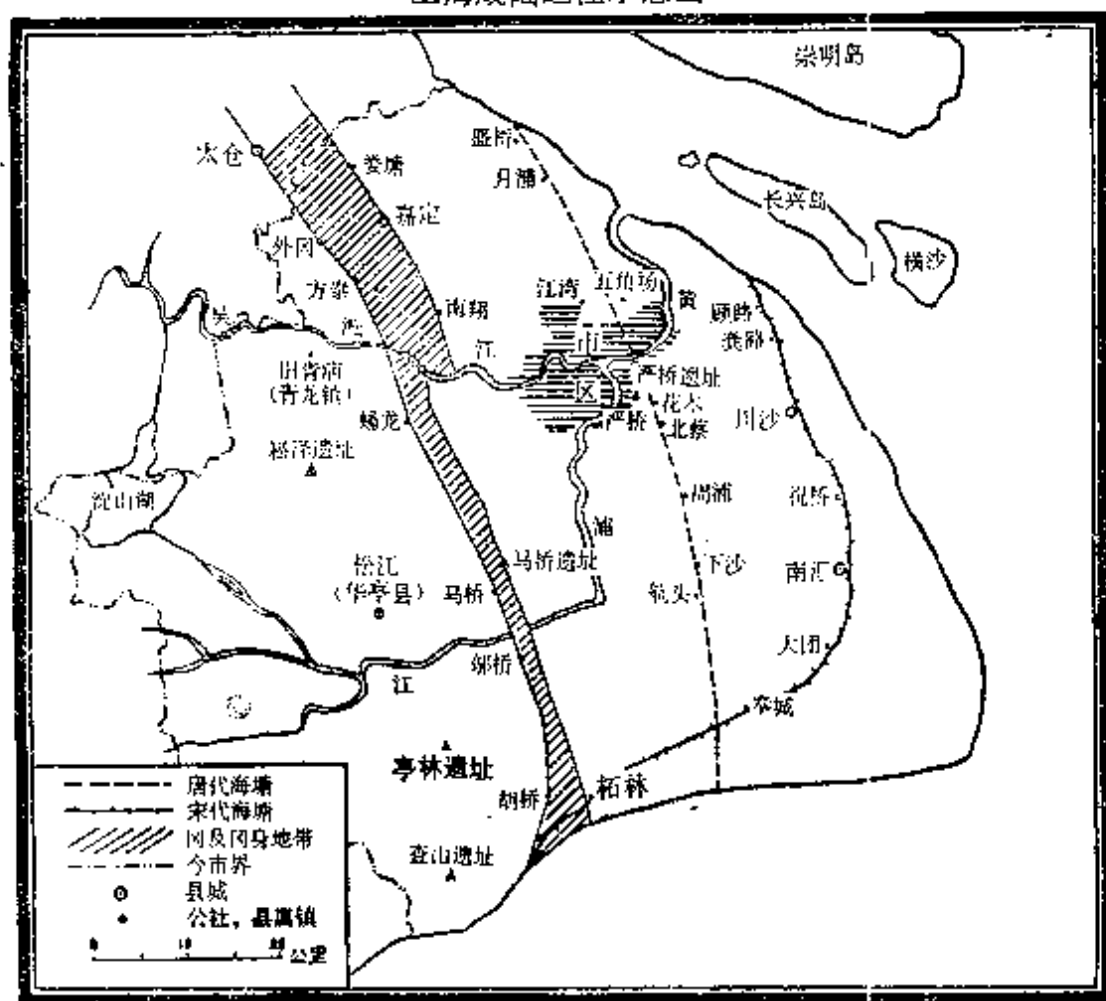
上海成陆过程示意图
