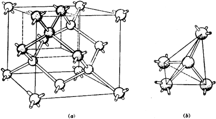
图 1.1.4 锗晶体结构示意图
