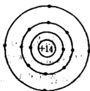
图 1.1.1 硅原子模型
