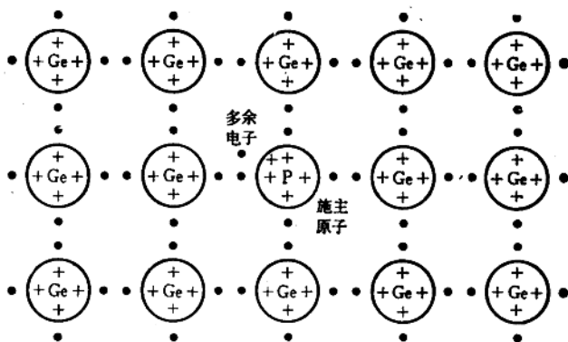
图 1.1.7 锗晶体中掺入少量磷原子的结构图
