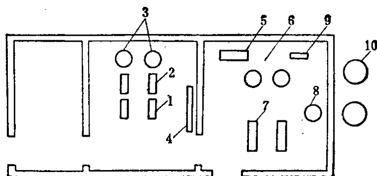
图 1-4 双级压缩机房布置
