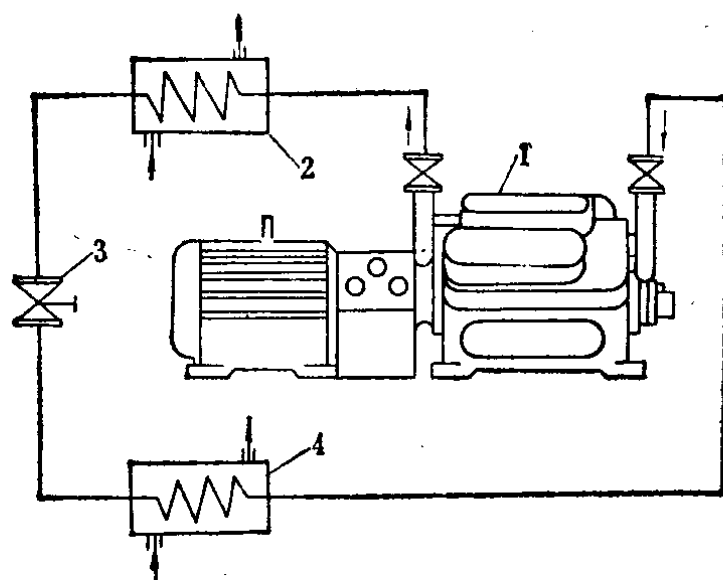
图 1-5 氨制冷原理图
