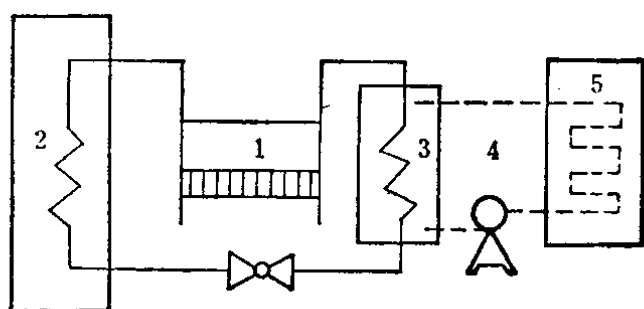
图 1-6 盐水冷却式制冷示意图
