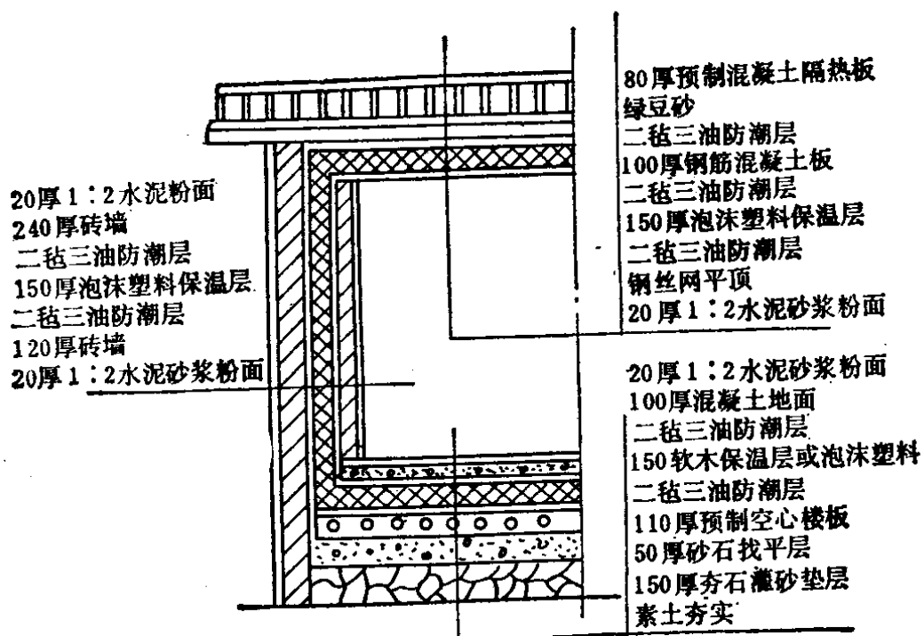
图 1-3 冷藏库库房的保温结构示意图
