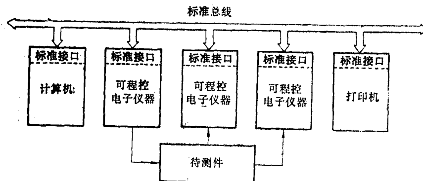
图1-0-3 现代自动测试系统
