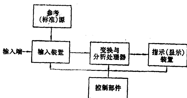
图1-0-2 测量被测量的量值的电子仪器的基本组成
