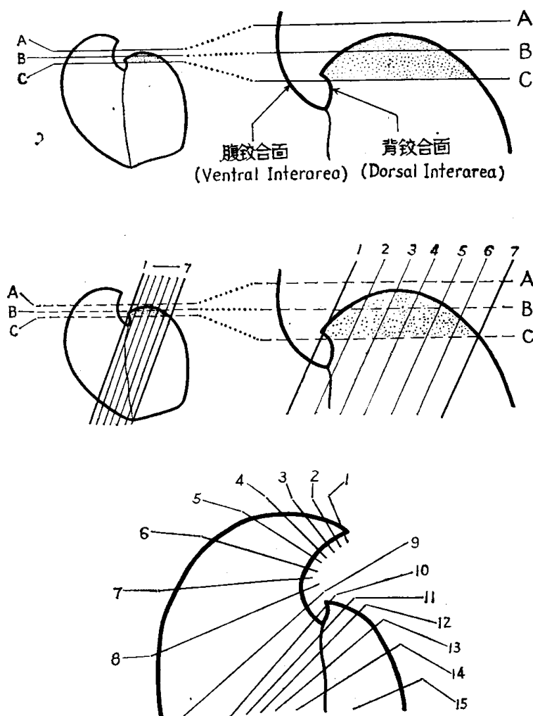
插图 2 喙部强烈弯曲的贝体系统横、斜切面的磨制方位示意图
