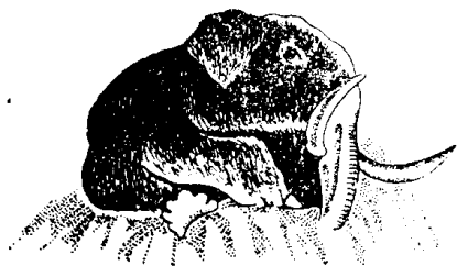
图 I 1-1 西伯利亚冻土层中发现的猛犸象化石
