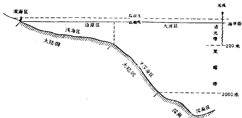
图 I 1-4 海洋环境的主要分区
