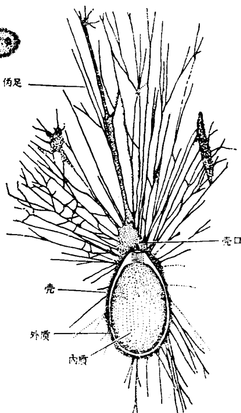
图 I 2-1-2 现代的有孔虫 Allogromia
