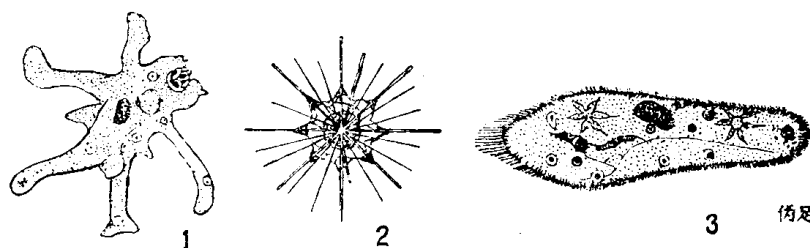
图 I 2-1-1 现代原生动物的某些类别
