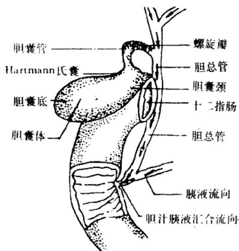
图2 胆囊示意图
