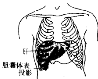
图1 胆囊的位置
