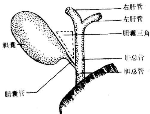
图 3 胆道模式图
