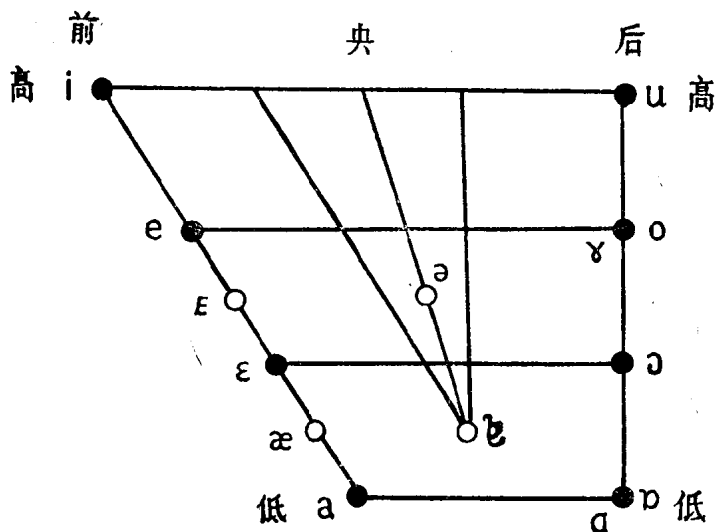
元音图
