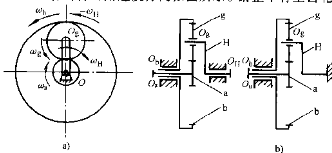
图 2-1 行星齿轮传动及其转化机构
