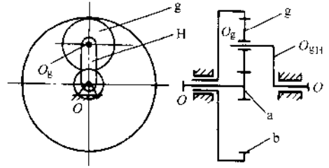
图 1-1 周转轮系
