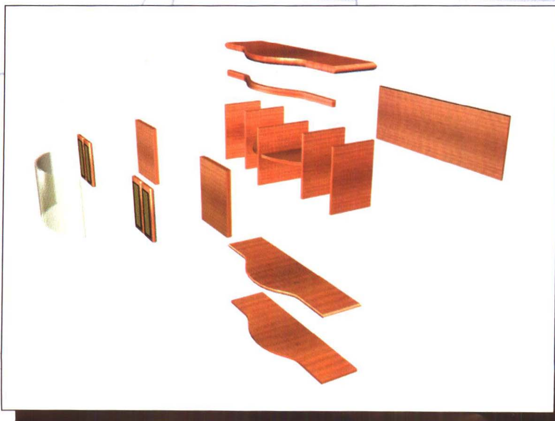
▼ 矮柜结构图
