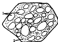
图 1-6 砾岩
