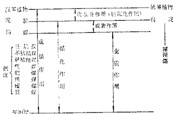
图 1-7 成煤过程划分示意图
