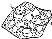
图 1-5 角砾岩
