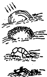
图 1-1 岩石的风化过程示意图
