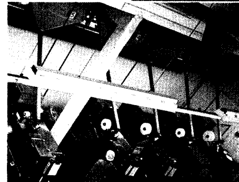
茶叶小包装自动化加工
