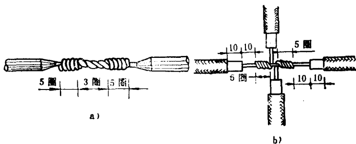
图1-6 单芯导线绞接联接
