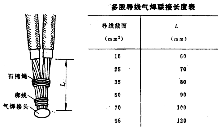
图1-5 多股导线气焊接头
