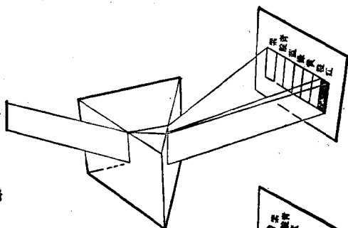
(a) 红地毯的光谱
