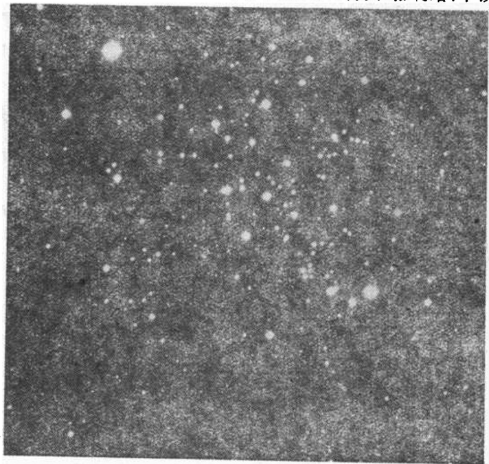
图 1-3 夜空的一部分。“被广阔空间分隔的孤立的物体。”
