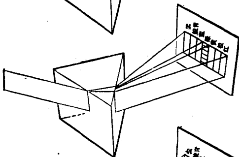
(a) 红地毯的光谱
