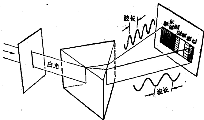
图 1-1 玻璃棱镜将白光变成基本色光谱。不同的颜色分别与不同的波长相对应。
