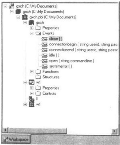
图 1-2 系统视图窗口
