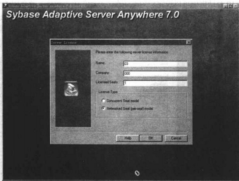
图 1-13 注册信息
