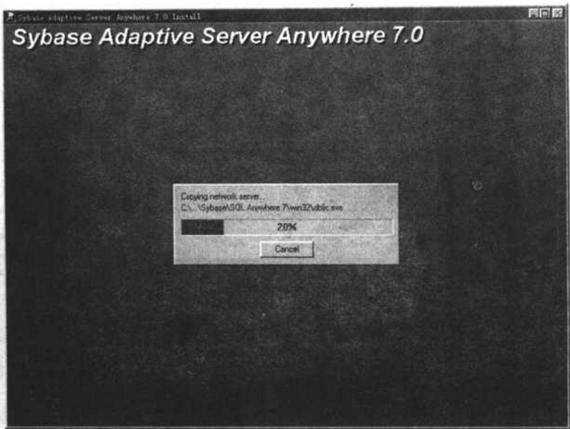
图 1-12 复制文件
