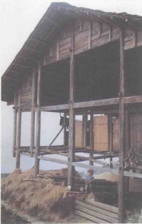
Casa de madera ganlan chuandou
