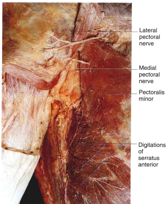
Fig. 2.7 Pectoralis minor.
