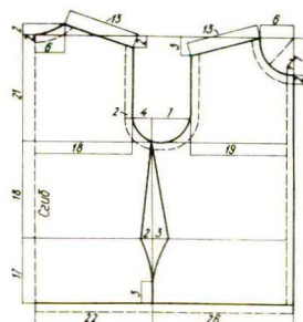
Спинка 1 дет
