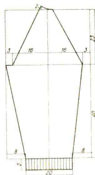
Рукав 2 дет.
