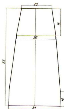
Спинка 1 дет. Перед 1 дет.
