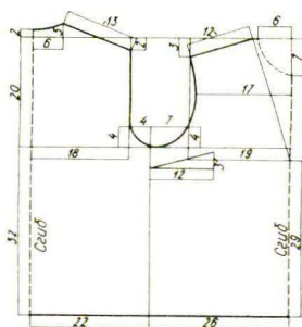
Спинка 1 дет. Перед 1 дет.
