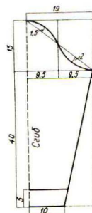
Рукав 2 дет.
