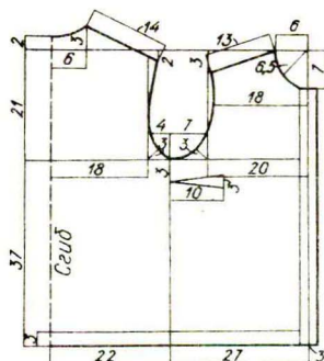
Спинка 1 дет. Перед 2 дет.
