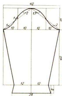
Рукав 2 дет.
