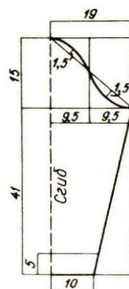
Рукав 2 дет.
