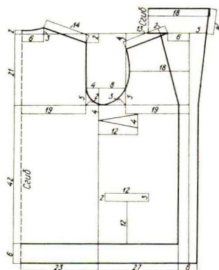
Спинка 1 дет. Перед 2 дет.
