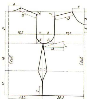
Спинка 1 дет. Перед 1 дет.
