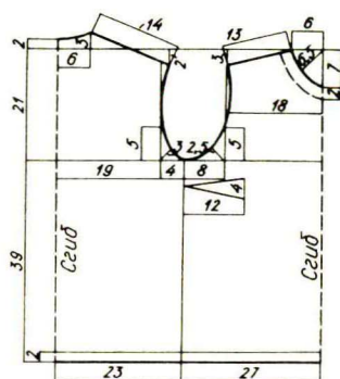
Спинка 1 дет. Перед 1 дет.
