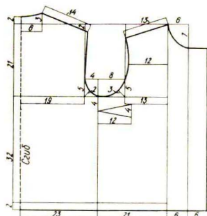
Спинка 1 дет. Перед 2 дет.
