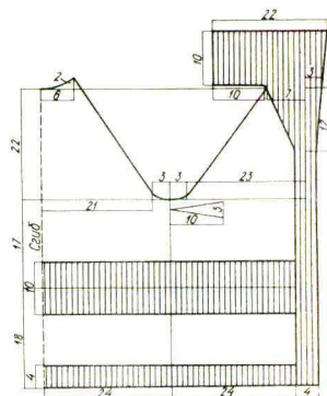
Спинка 1 дет.
