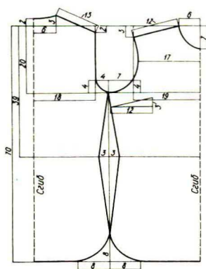
Спинка 1 дет. Перед 1 дет.
