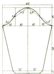
Рукав 2 дет
