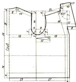
Спинка 1 дет.
