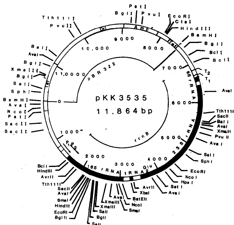
FIG. 1. Plasmid pKK3535 (1).
