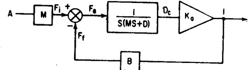
Fig. 3. Simple servoed accelerometer.
