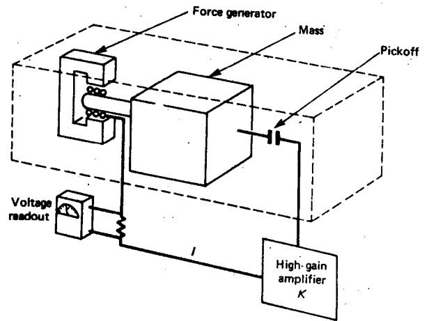
Fig. 3. Simple servoed accelerometer.
