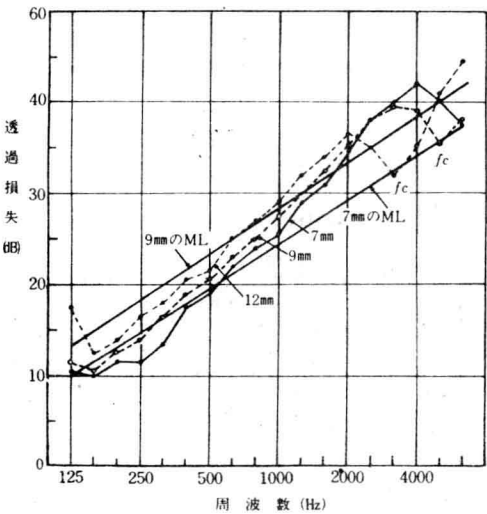
11. 石こうボードの遮音特性
