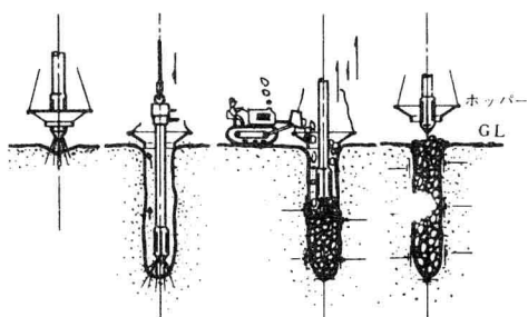
(a) 貫入開始 (b) 貫入完了 (c) 骨材充填締め (d) 締め完了
