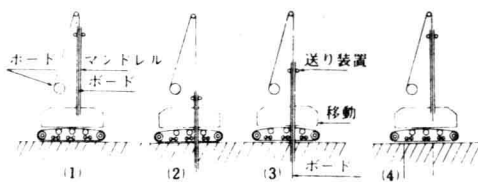
12. ペーパー・ドレーン工法の施工順序 （マンドレル打設法）
