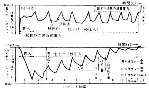
7. パイロ・コンポーザーによる施工管理記録
