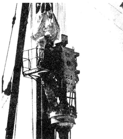
15. 材料の投入(ケミコパイル工法)
