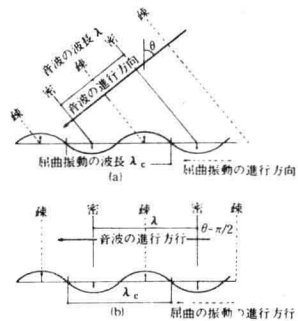
9. コインシデンス効果の発生機構
