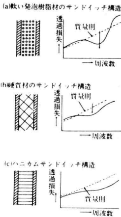
4. サンドイッチボードの遮音特性
