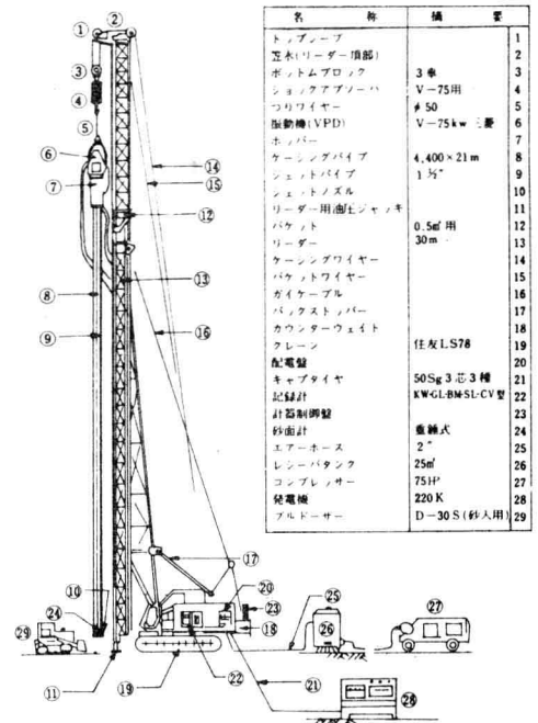
6. パイロ・コンポーザー施工機
