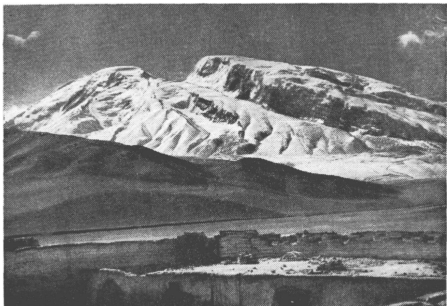
Высочайшая вершина Куньлуня Музтагата.
