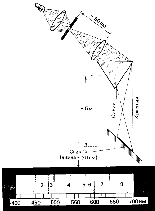
Рис. 1.1. Разложение белого света в спектр:
