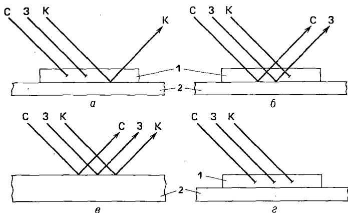
Рис. 1.6. Цвет непрозрачных предметов:
