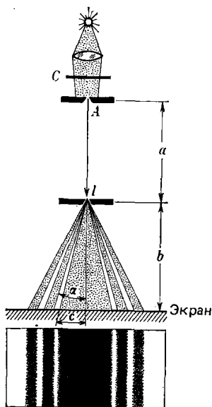
Рис. 1.5. е Ограничение пучка света узкой щелью. Схема установки и участок изображения, получающегося на белом экране при огибании светом краев щели:
