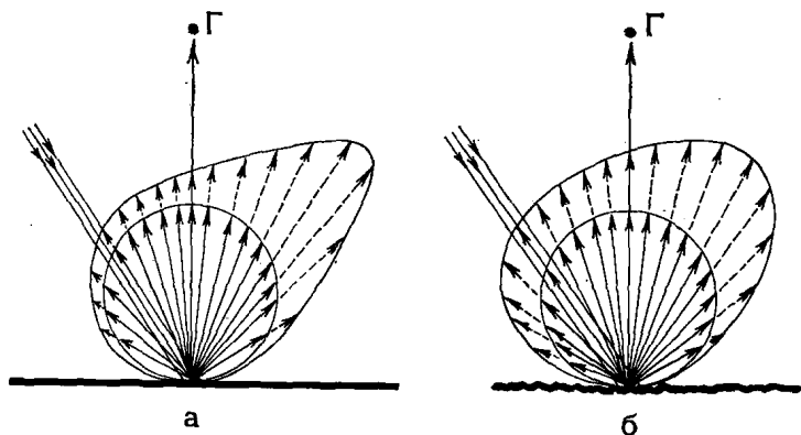
Рис. 1.10 Отражение света от поверхности мелованной (а) и немелованной (б) бумаги:
