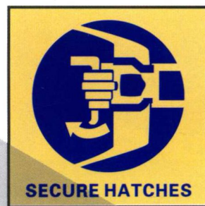
关紧舱门
