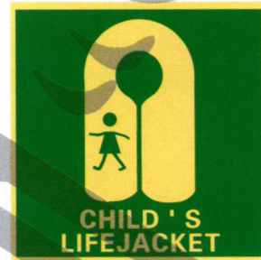
儿童救生衣
