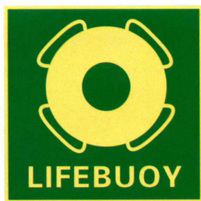
救生圈
