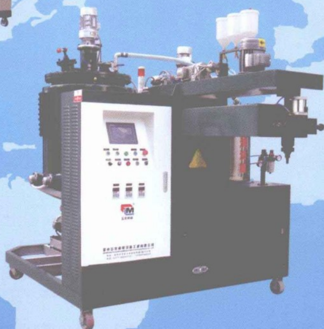
CPU20FS-G系列 聚氨酯可加色浆弹性体浇注机 (高配置) CPU20FS-G SERIES PU COLOR PASTE ADDABLE ELASTOMER CASTING MACHINE (HIGH CONFIGURATION)
