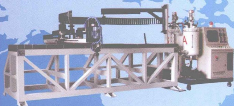
PU20F-AR系列 全自动数控三维异形密封条浇注机 FULL-AUTO NUMERICAL CONTROL 3D POURING MACHINE FOR SHAPED SEALING STRIP
