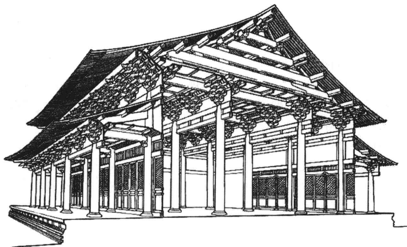
图 0 - 3 《营造法式》中大木作殿堂结构示意图
