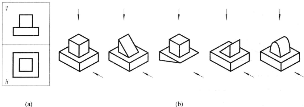
图 1-14 形体的两面投影
