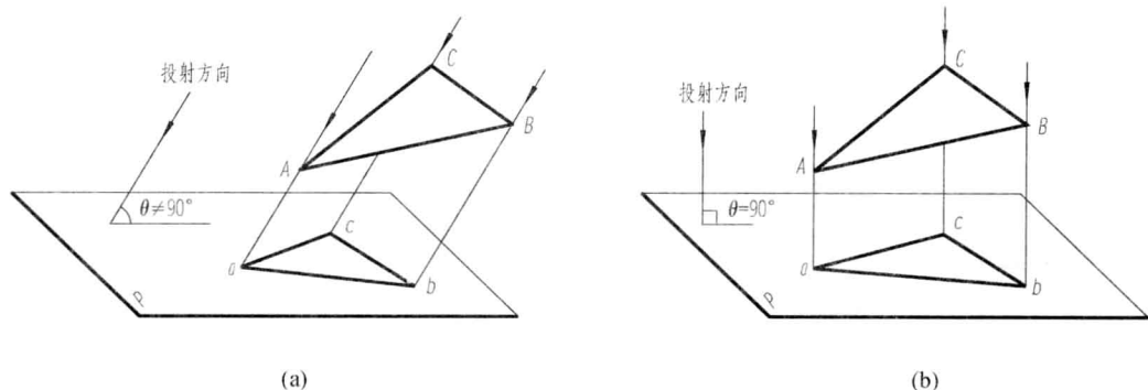
图 1-3 平行投影法 (a) 斜投影法; (b) 正投影法
