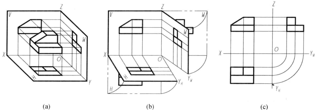
图 1-9 多面正投影法
