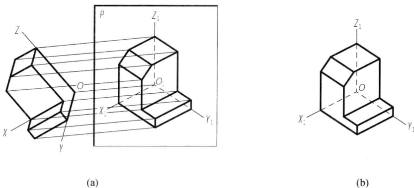
图 1-10 轴测投影法
