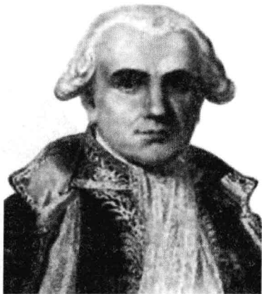
图 0-1 加斯帕·蒙日
