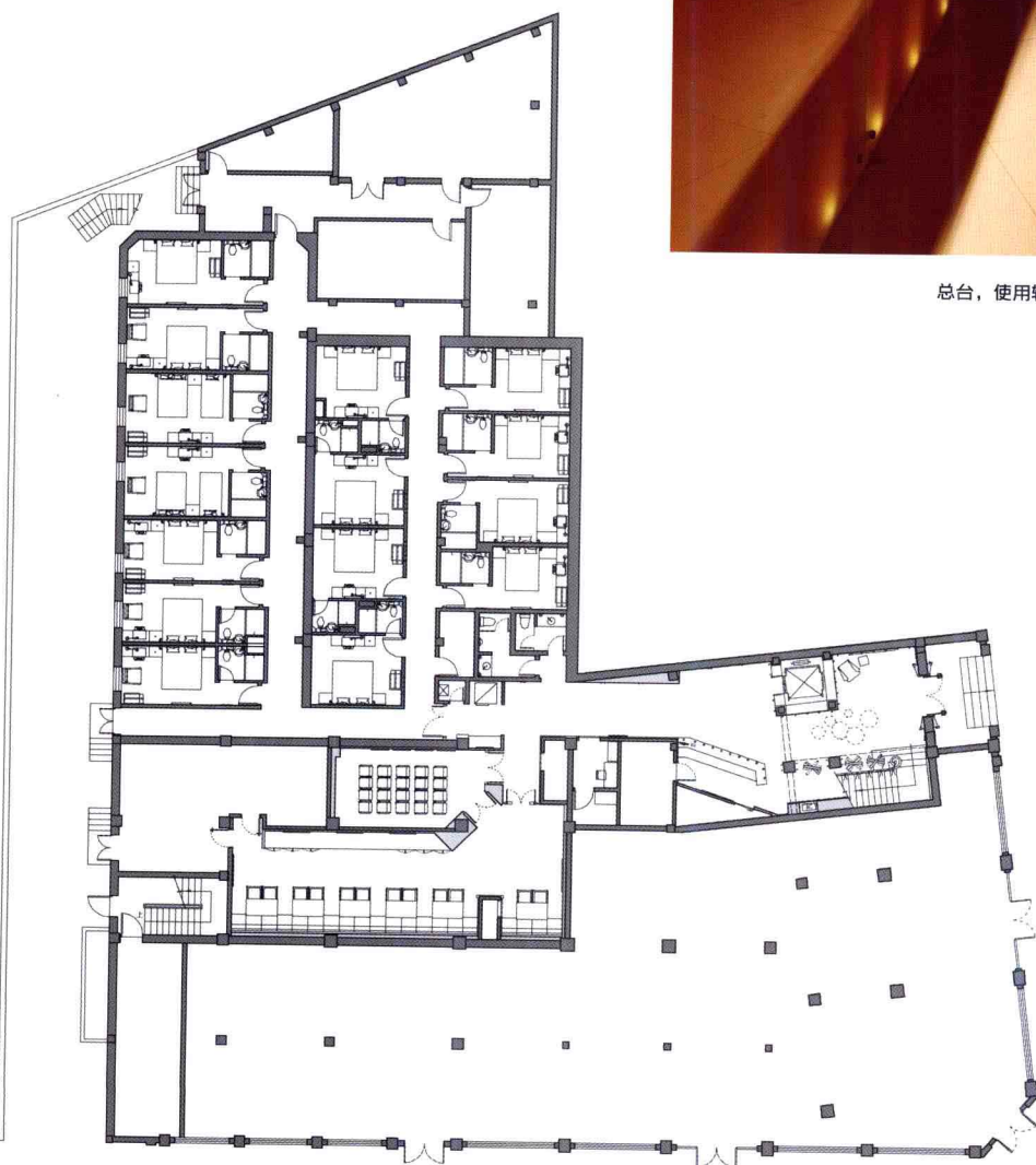
平面图
