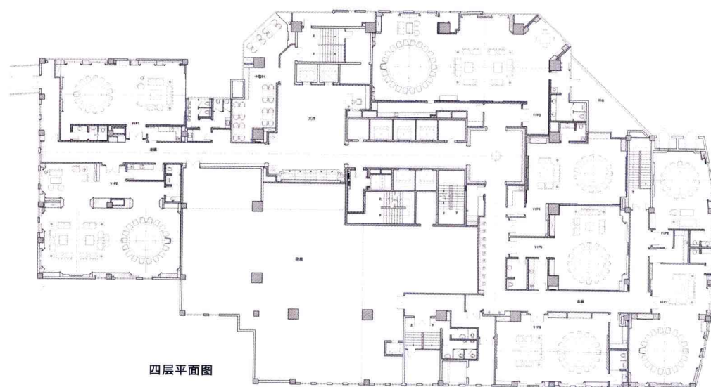
四层包间
