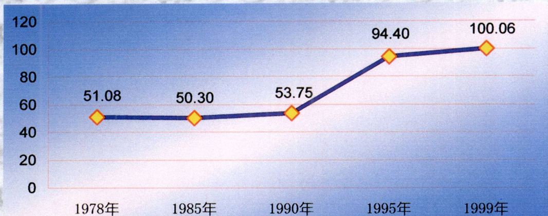
公路密度(公里/百平方公里)
