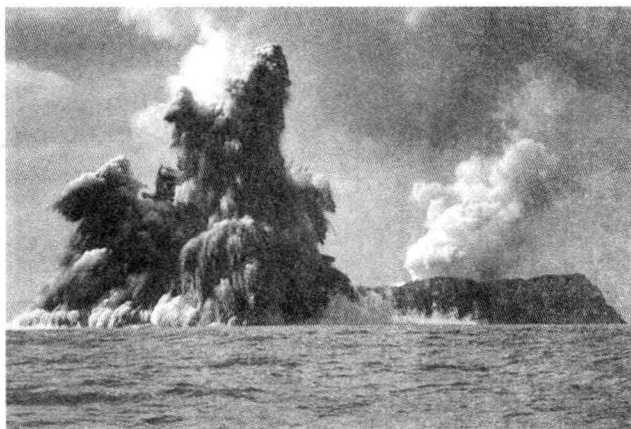
海底火山爆发
