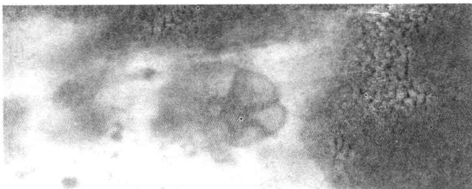
在一批形成于白垩纪时期的琥珀中发现了稀有的海洋
