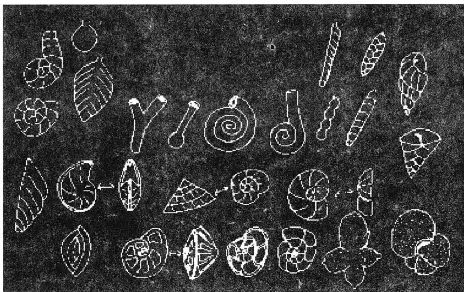
有孔虫的绘图
