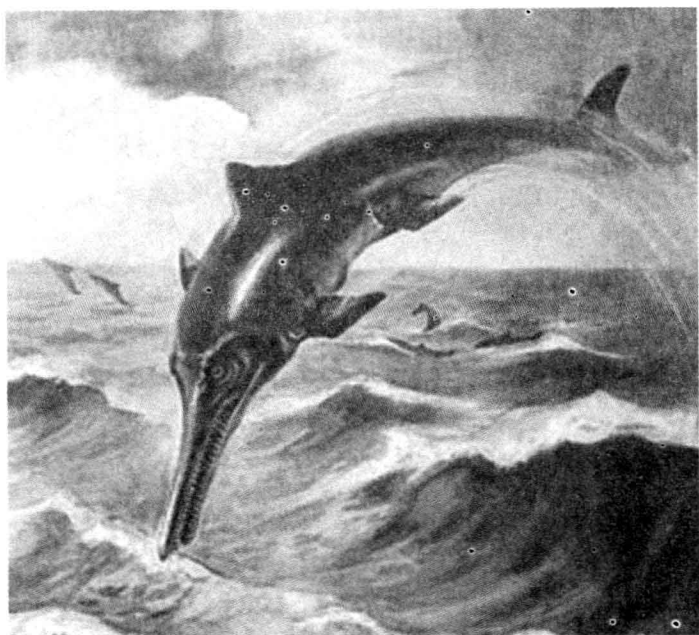
白垩纪时期的海洋
