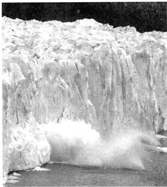
冰川时代的冰川
