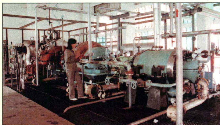
運轉在鎮海化肥廠獲國家金牌獎的年產52萬噸尿素裝置的CO 2 離心壓縮機
