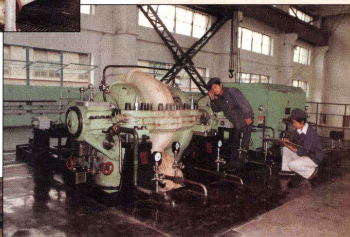
運轉在蘭州煉油廠的榮獲國家銀質獎的2MCL457離心壓縮機
