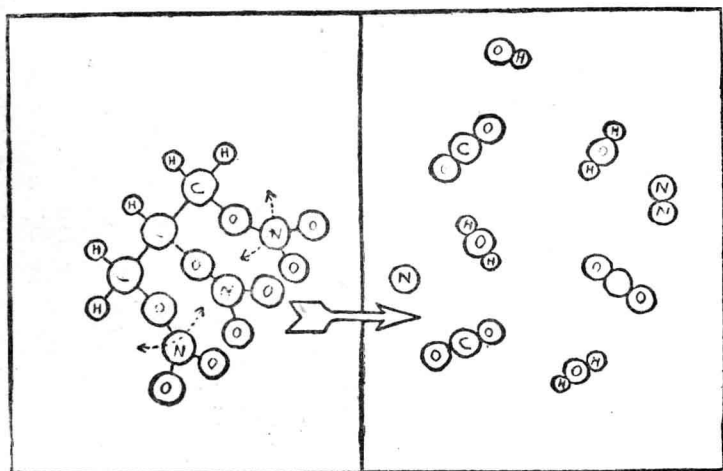
圖2. 三硝酸丙三醇 (glyceryl trinitrate) 的介穩分子之放熱分解，換句話說就是硝化甘油的爆炸。這時強烈的熱振動使氧原子（預先被氮原子隔離而孤立者）包圍碳原子和氫原子，結果全分子破裂而解放內部的能。
