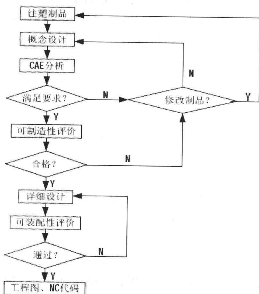
图 1-1 设计流程图
