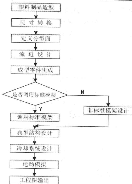
图 1-2 模具结构详细设计的流程图
