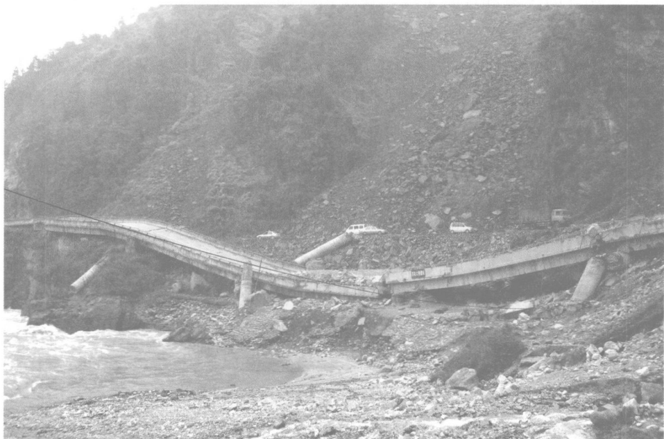
在大地震中倒塌的百花大桥。
