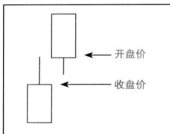
• 图1-2 高开
