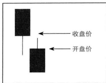
• 图1-5 低开
