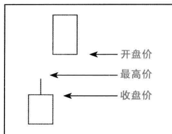
• 图1-3 跳空高开
