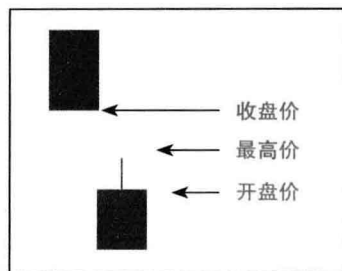
• 图1-6 跳空低开
