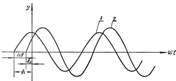
图 1-2 具有相位差 \Delta\varphi 的两个同频的简谐振动 1-y_1 = A_1 \sin(\omega t + \varphi_1) , 2-y_2 = A_2 \sin(\omega t + \varphi_2)
