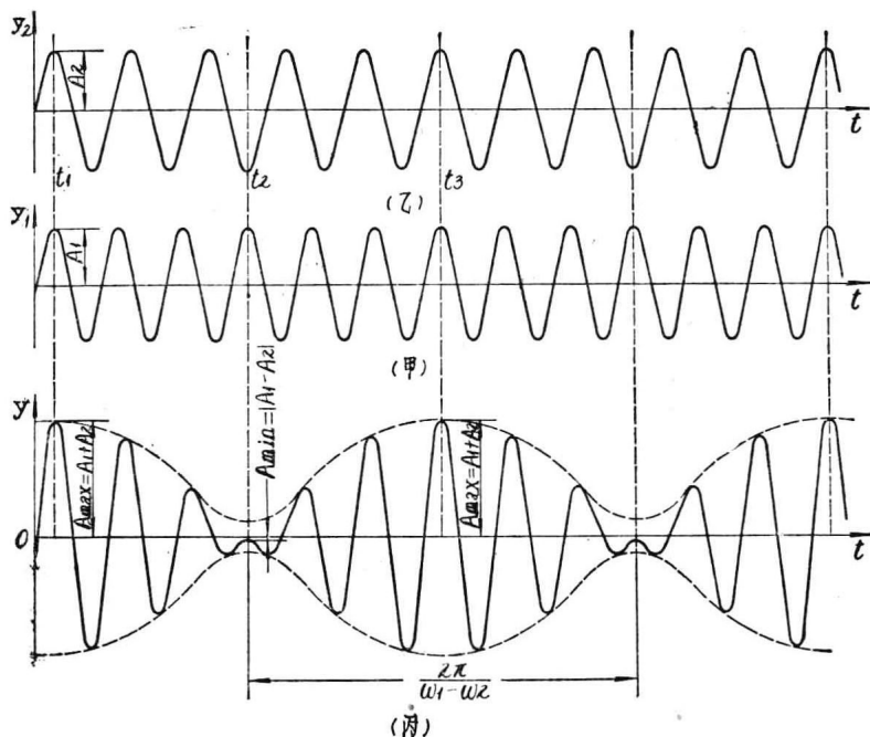
图 1-8 拍
