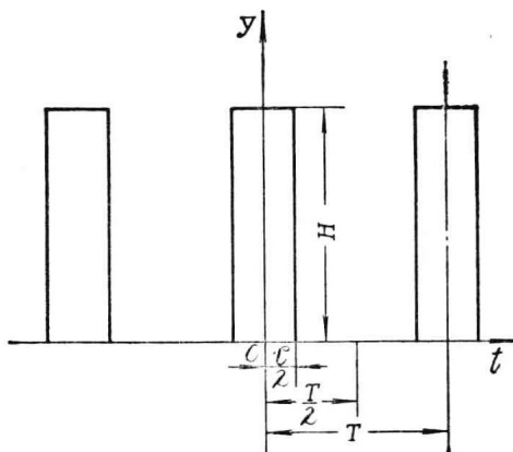
图 1-9 方脉冲波
