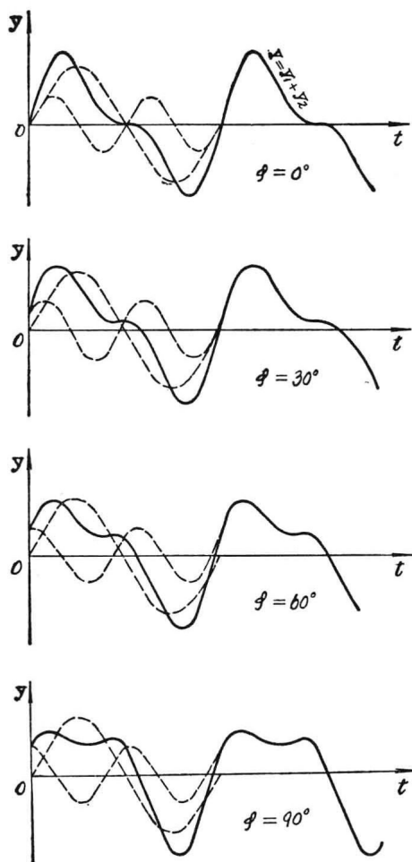
图 1-6 \omega_2 = \alpha\omega_1 时两个同方向简谐振动的合振动波形
