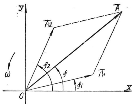
图 1-5 同向同频简谐振动的合成
