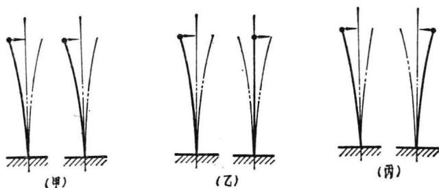
图 1-3 叶片振动时的相位差示意图
